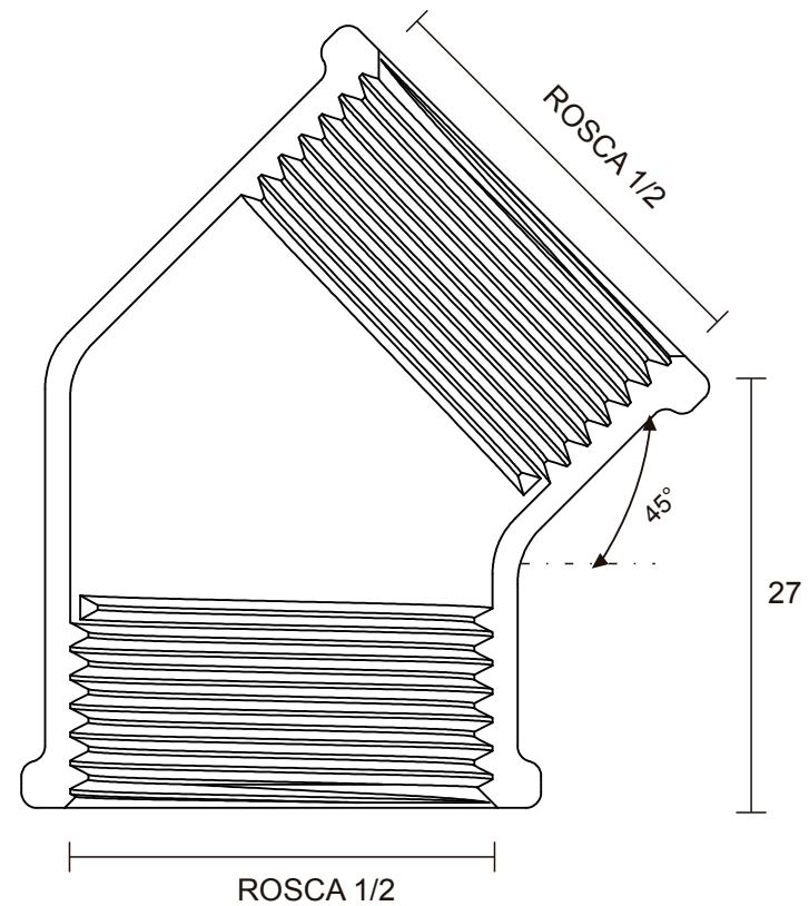
CORTE B-B
