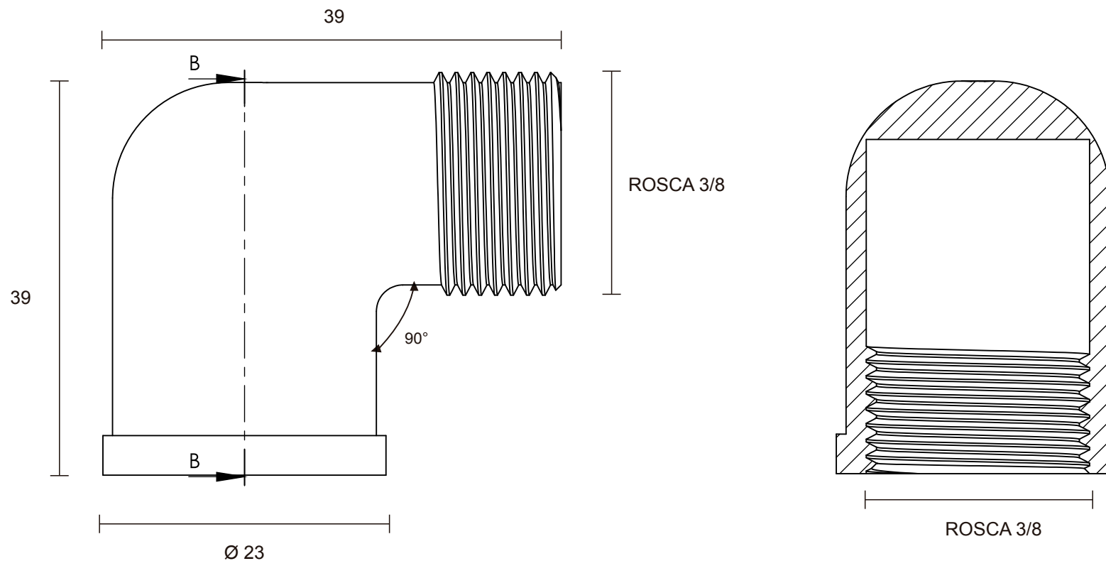
CORTE B-B
